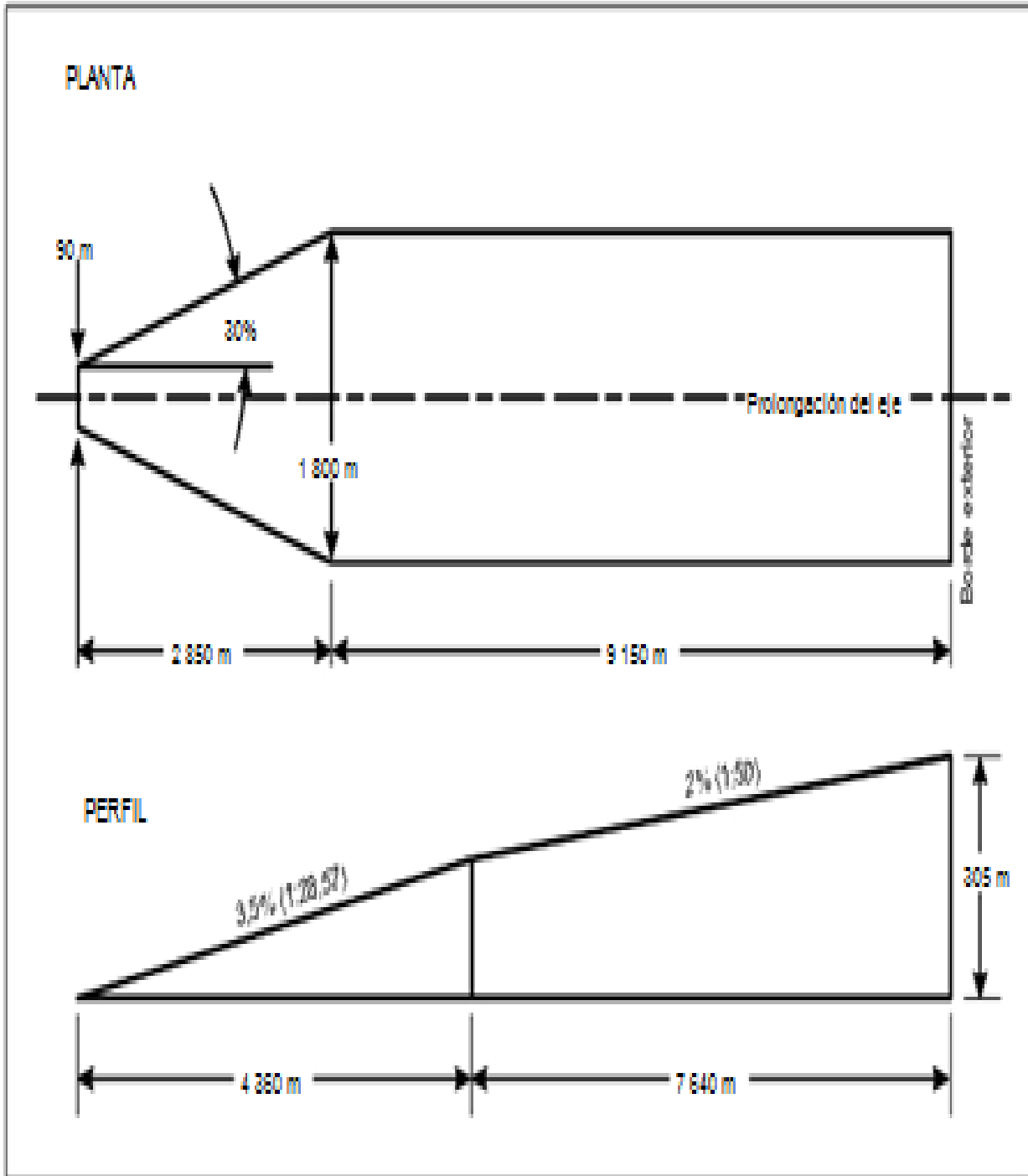
Figura 4-5. Superficie de ascenso en el despegue de la FATO en vuelo por instrumentos
