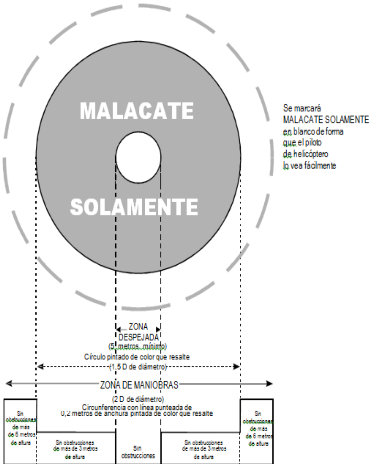
Figura 4-11. Área de carga y descarga con malacate a bordo de un buque
