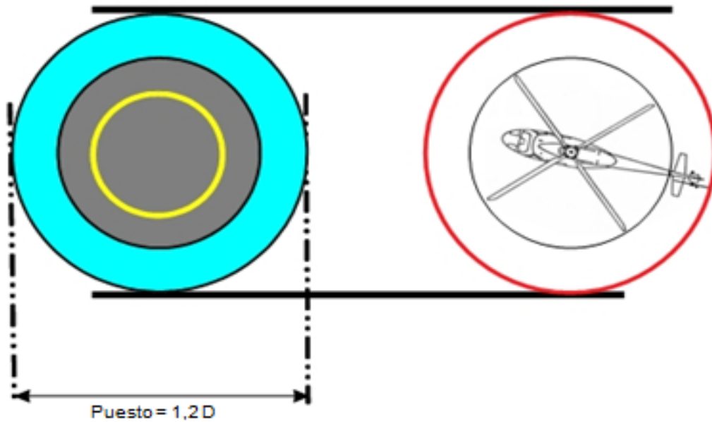
Figura 3-4. Puesto de estacionamiento de helicópteros
