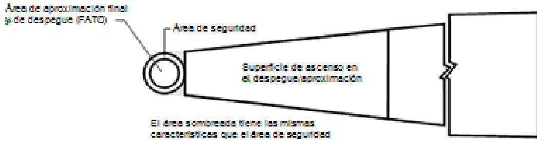
A. Área de aproximación final y de despegue de forma circular (aproximación-salida en línea recta)
