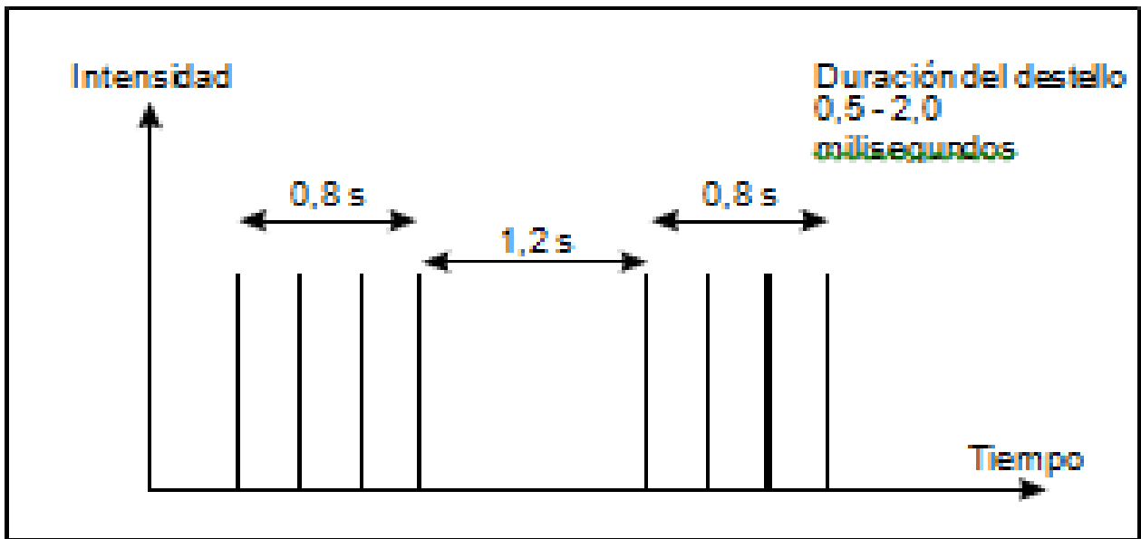
Figura 5-8. Características de los destellos de un faro de helipuerto
