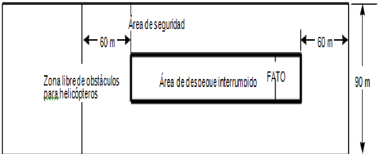
Figura 3-1. Área de seguridad de la FATO para aproximaciones por instrumentos
