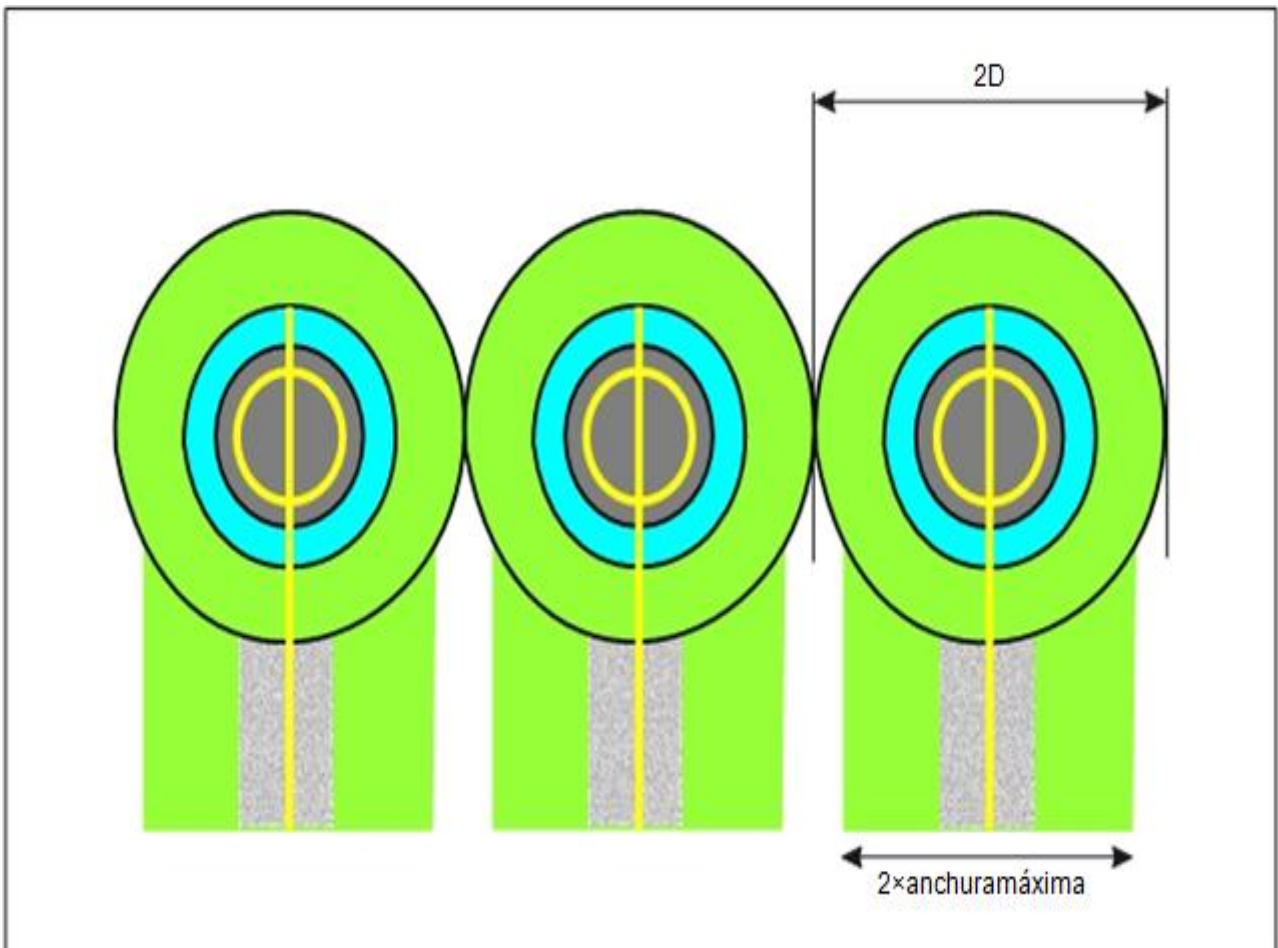
Figura 3-6. Puestos de estacionamiento de helicópteros diseñados para virajes estacionarios en rutas/calles de rodaje aéreo — operaciones simultáneas
