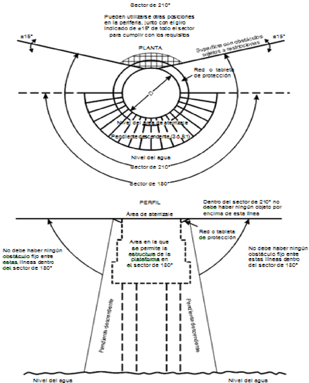
Figura 4-2. Sector despejado de obstáculos de una heliplataforma
