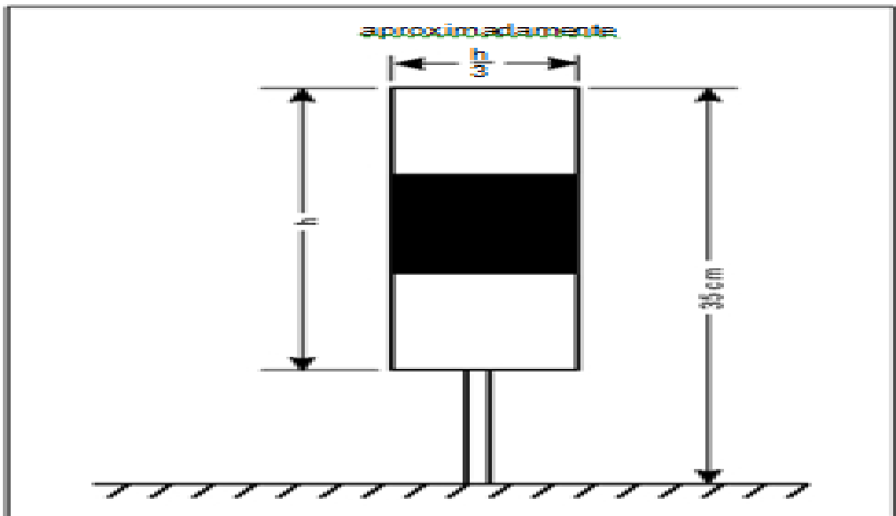
Figura 5-6. Baliza de calle de rodaje aéreo
