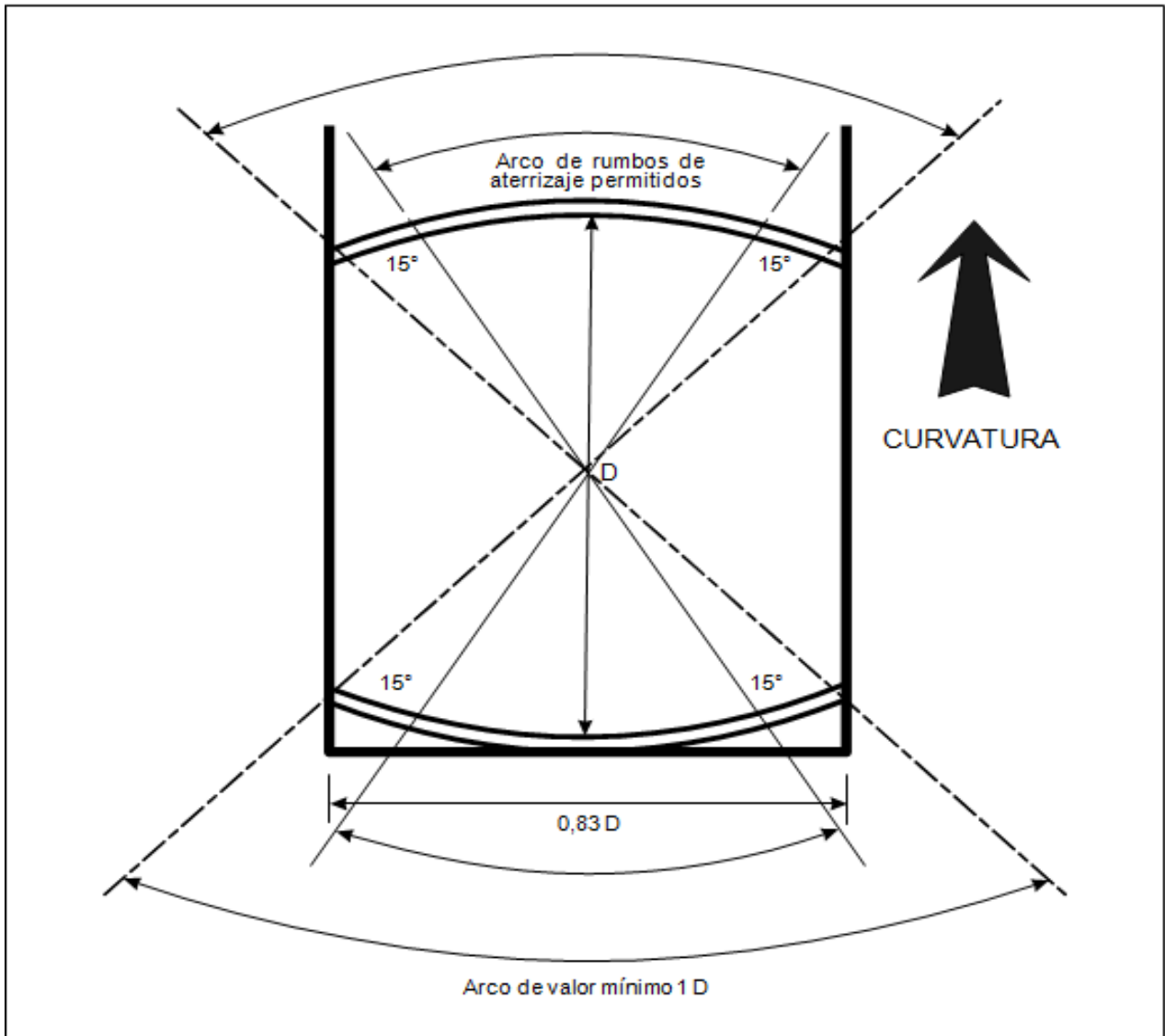
Figura 3-8. Rumbos de aterrizaje permitidos a bordo de un buque para operaciones con rumbos restringidos
