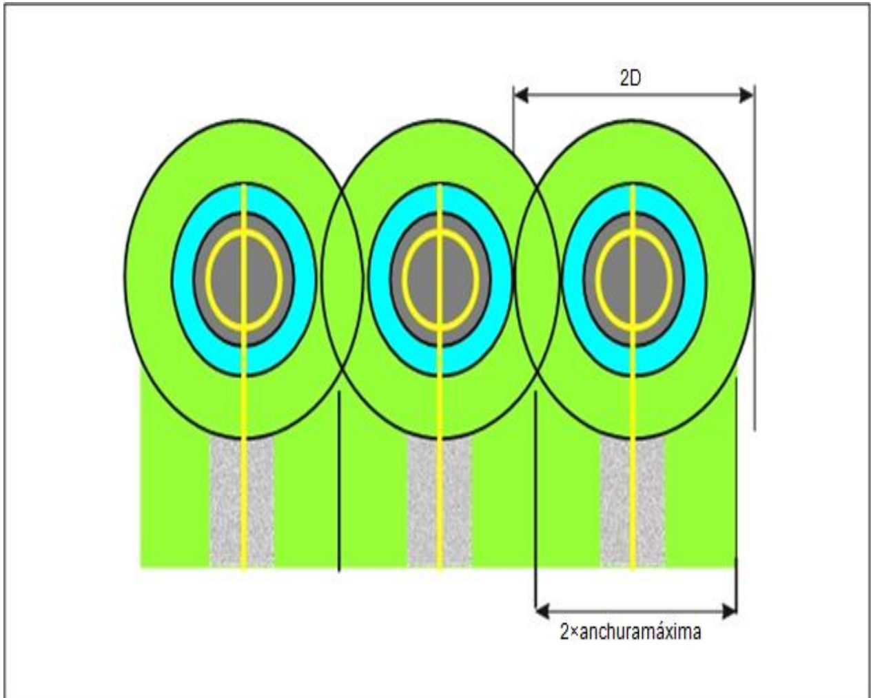
Figura 3-7. Puestos de estacionamiento de helicópteros diseñados para virajes estacionarios en rutas/calles de rodaje aéreo — operaciones no simultáneas
