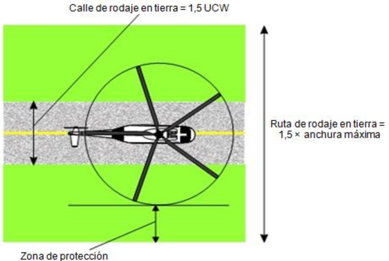
Figura 3-2. Ruta de rodaje en tierra
