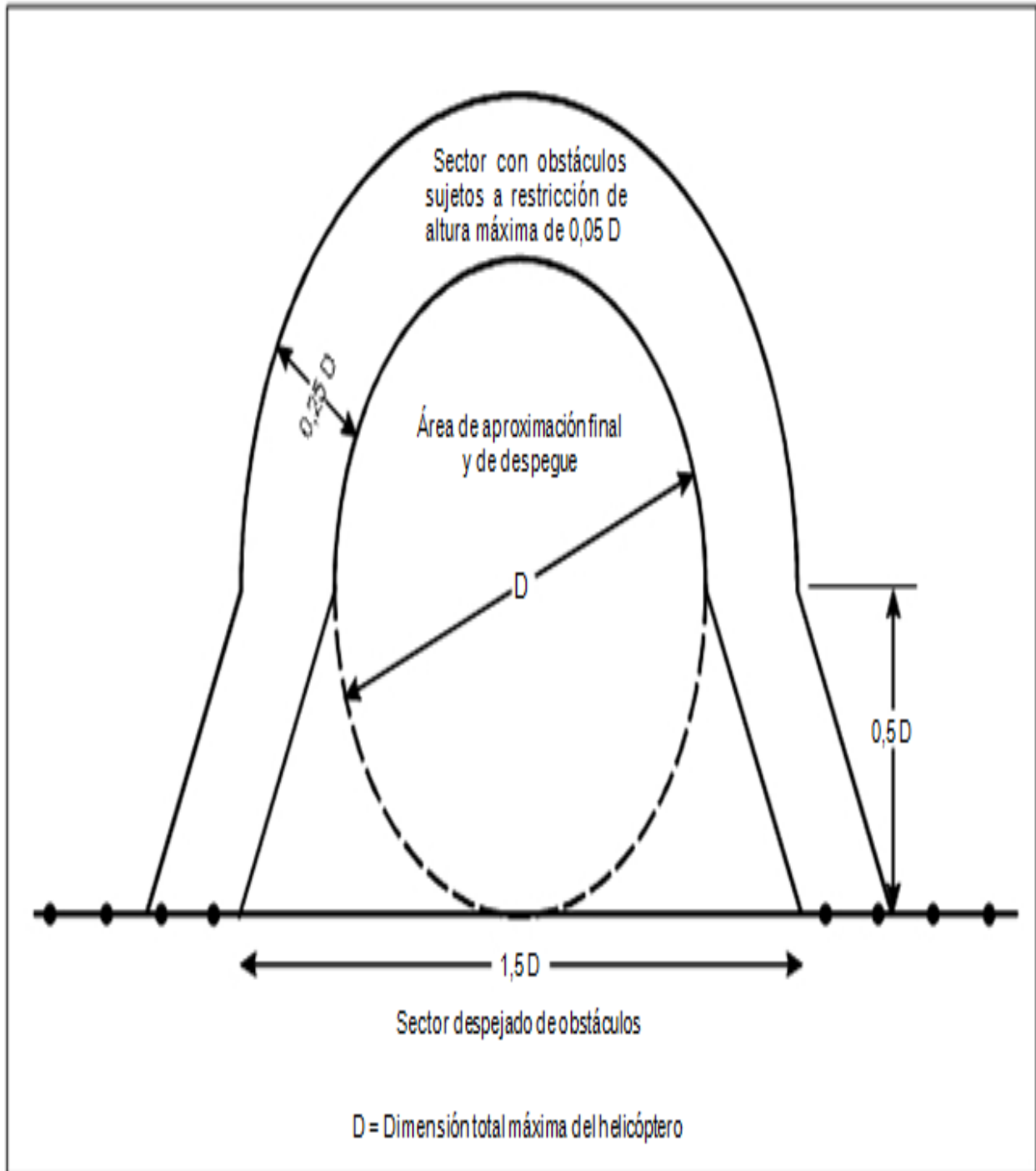
Figura 4-10. Superficies limitadoras de obstáculos en los helipuertos no construidos para fines especiales en el costado del buque
