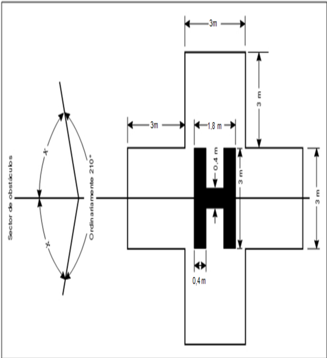
Figura 5-1. Señal de identificación de helipuerto (indicada con una cruz de hospital y orientada con el sector despejado de obstáculos)
