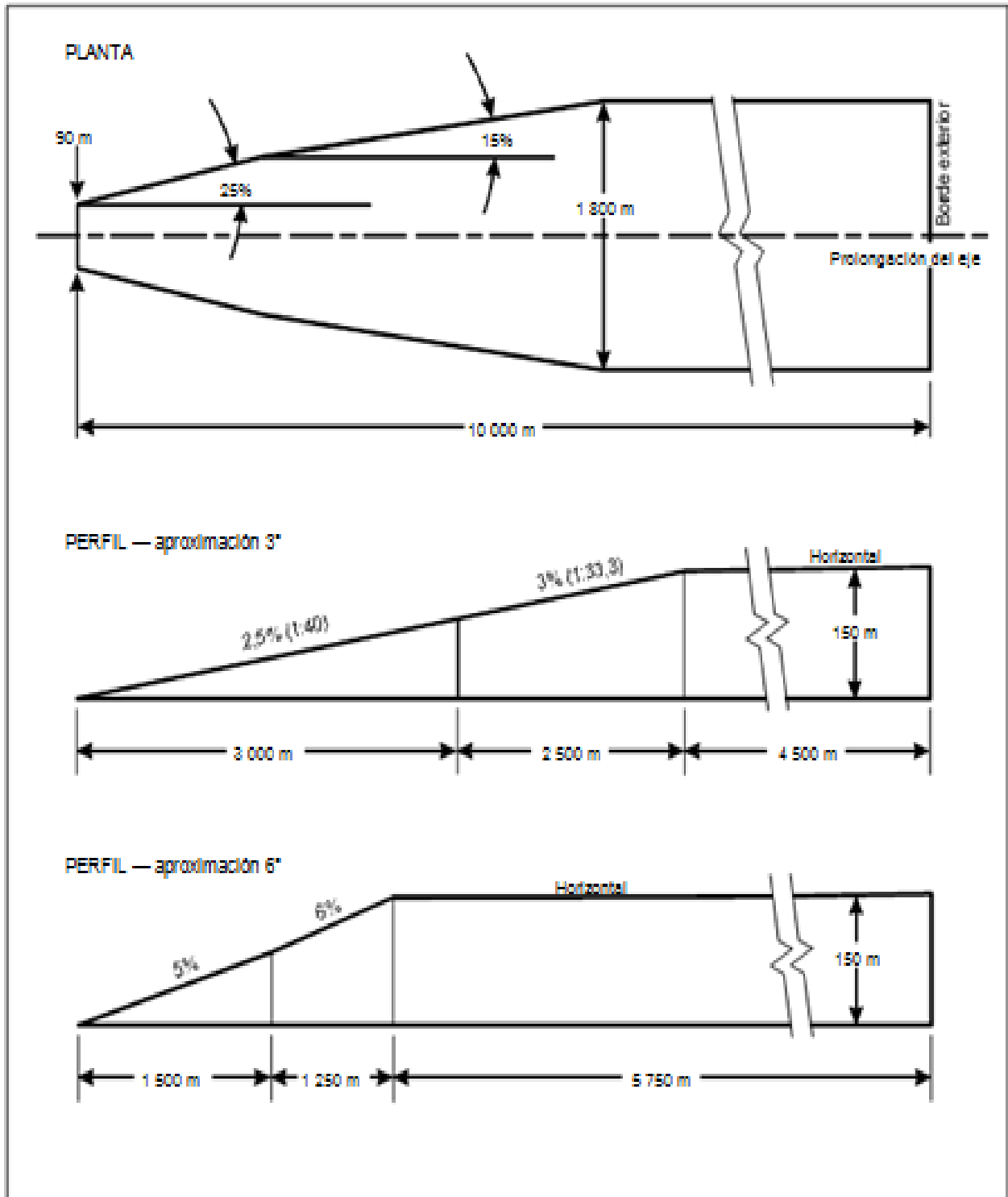
Figura 4-6. Superficie de aproximación de la FATO para aproximaciones de precisión
