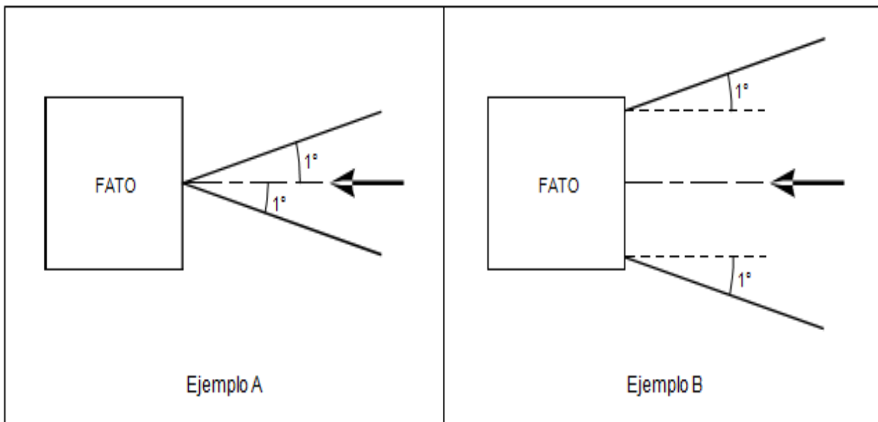
Figura 5-11. Divergencia del sector "derrota correcta"
