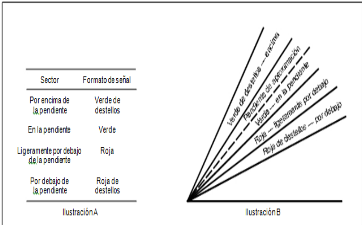
Figura 5-13. Formato de la señal HAPI
