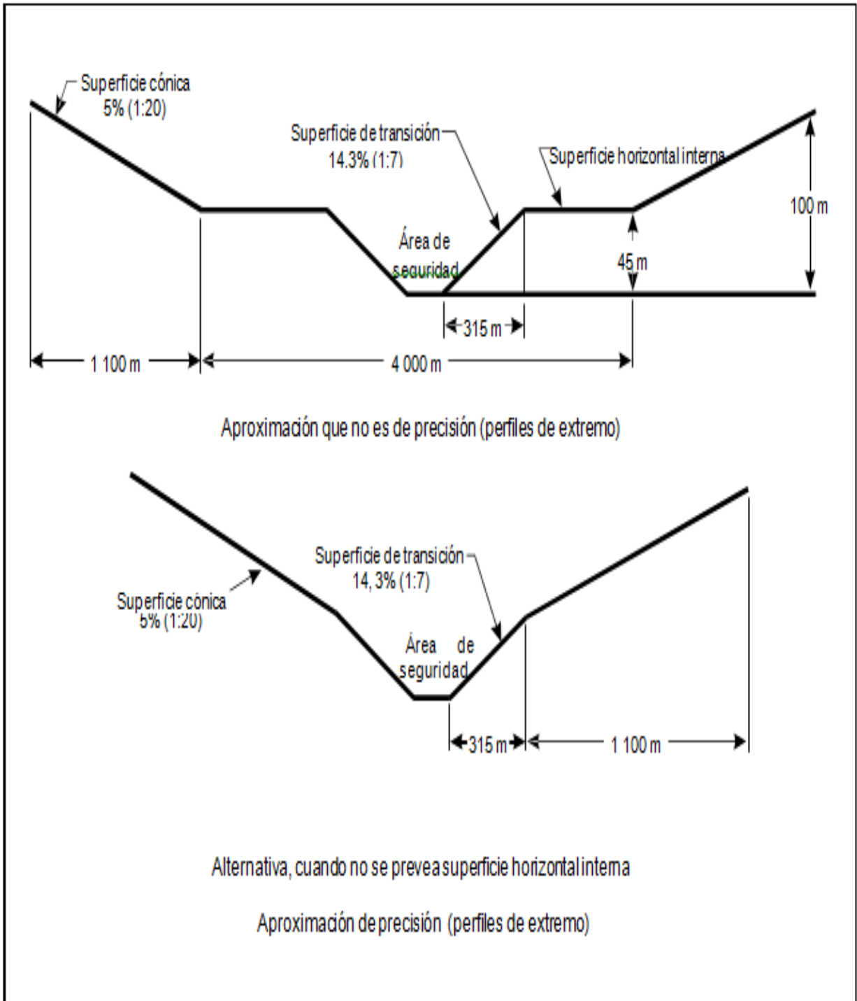
Figura 4-8. Superficies limitadoras de obstáculos de transición, horizontal interna y cónica
