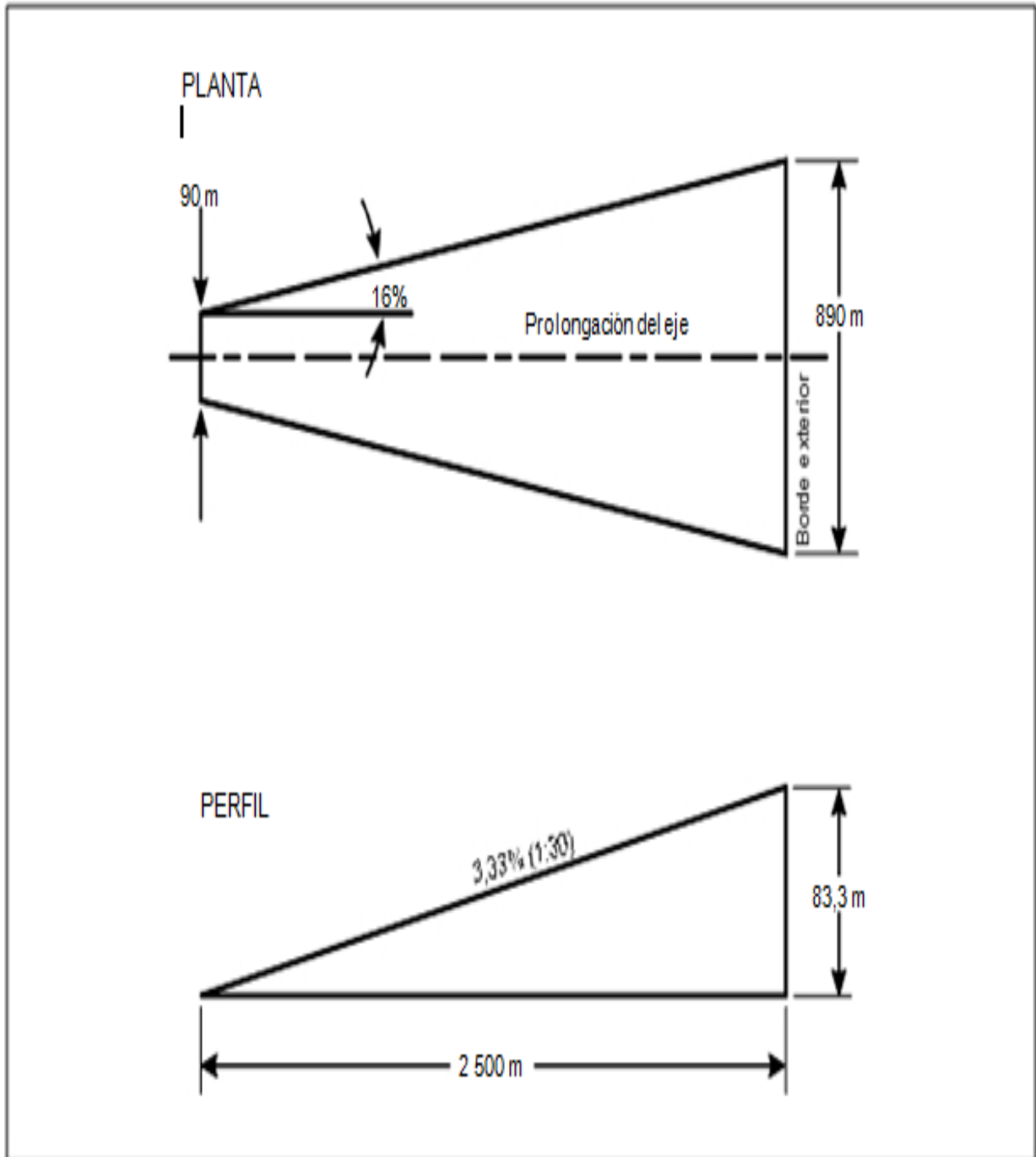
Figura 4-7. Superficie de aproximación de la FATO para aproximaciones que no sean de precisión
