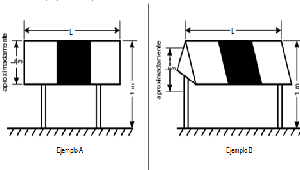
Figura 5-7. Baliza de ruta de desplazamiento aéreo
