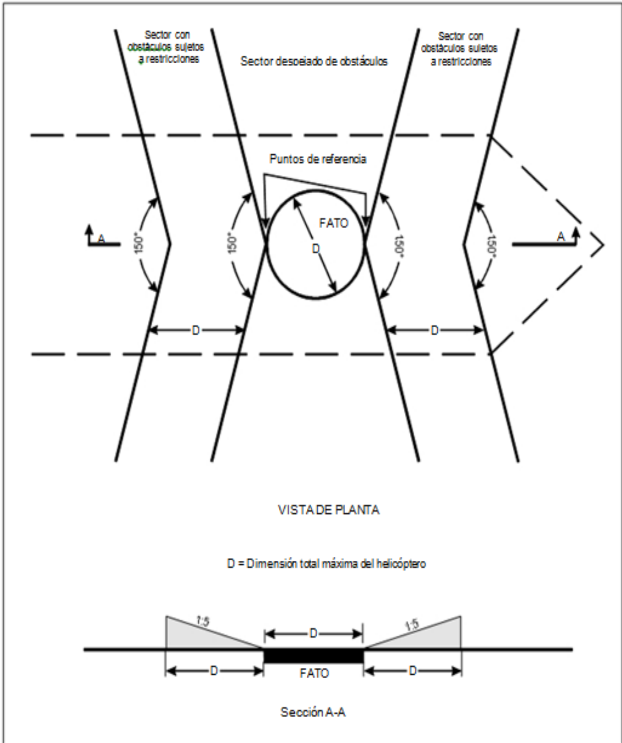
Figura 4-9. Superficies limitadoras de obstáculos en los helipuertos no construidos para fines especiales en el costado del buque
