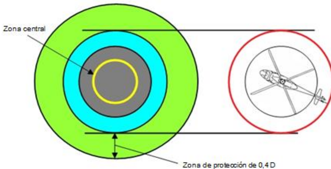
Figura 3-4. Puesto de estacionamiento de helicópteros
