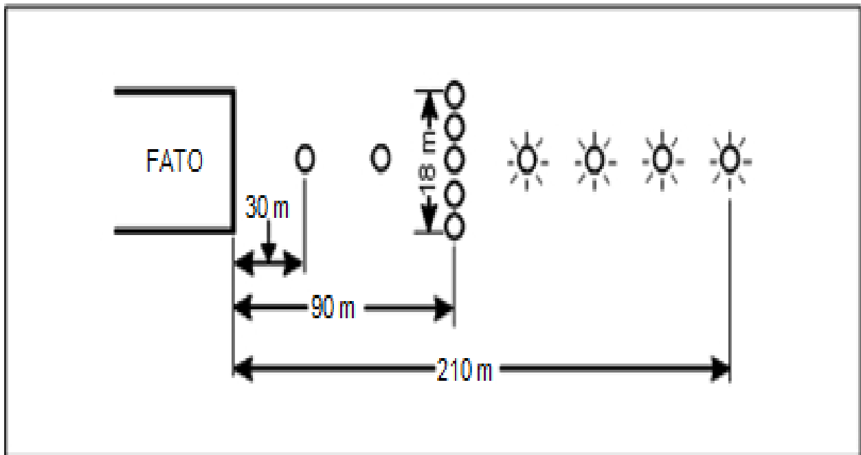
Figura 5-10. Sistema de luces de aproximación
